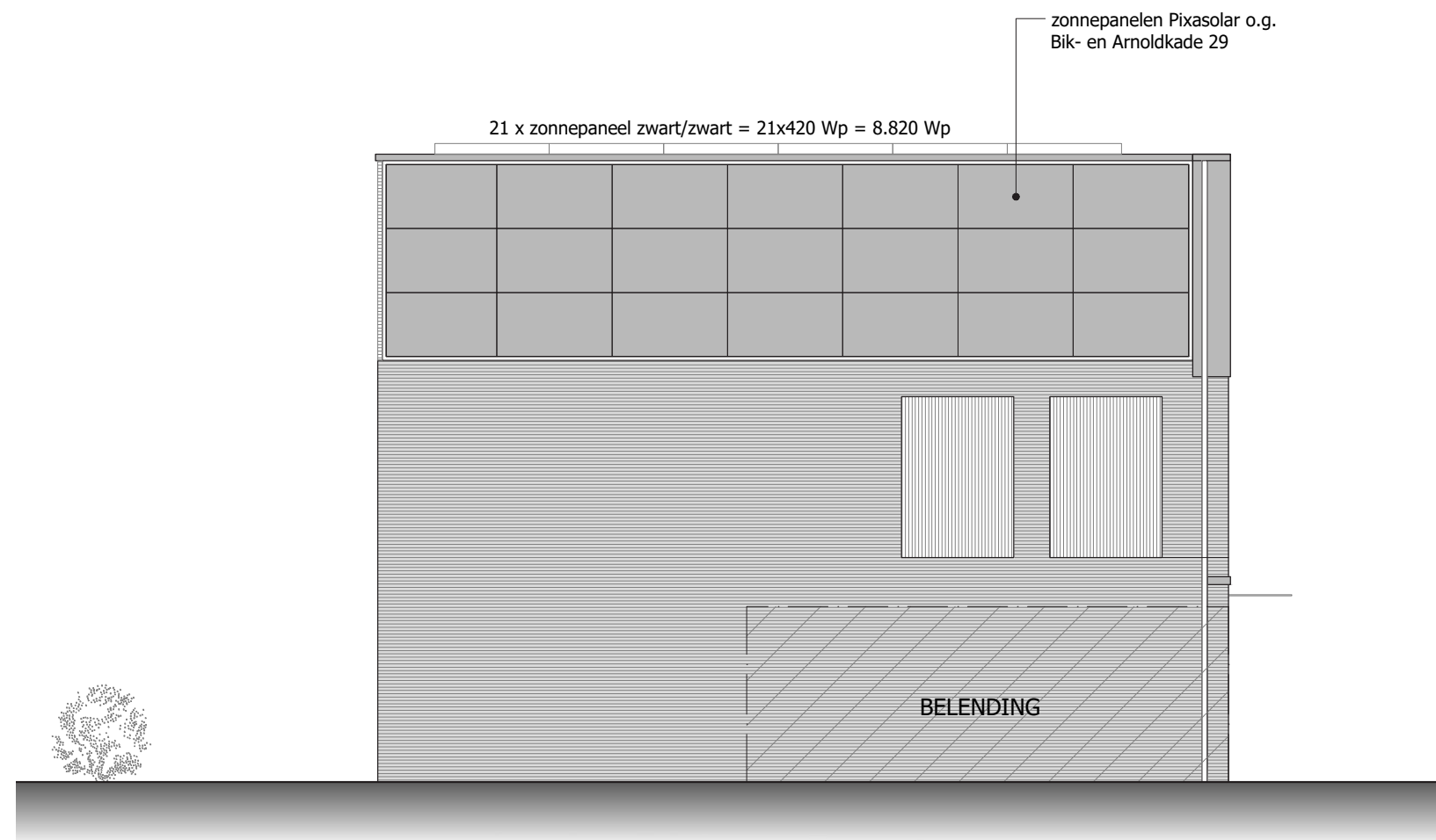
Linker zijgevel
