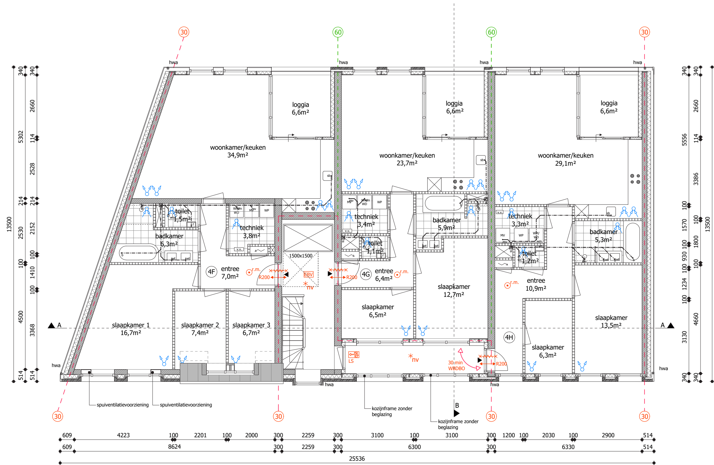
Tweede verdieping
