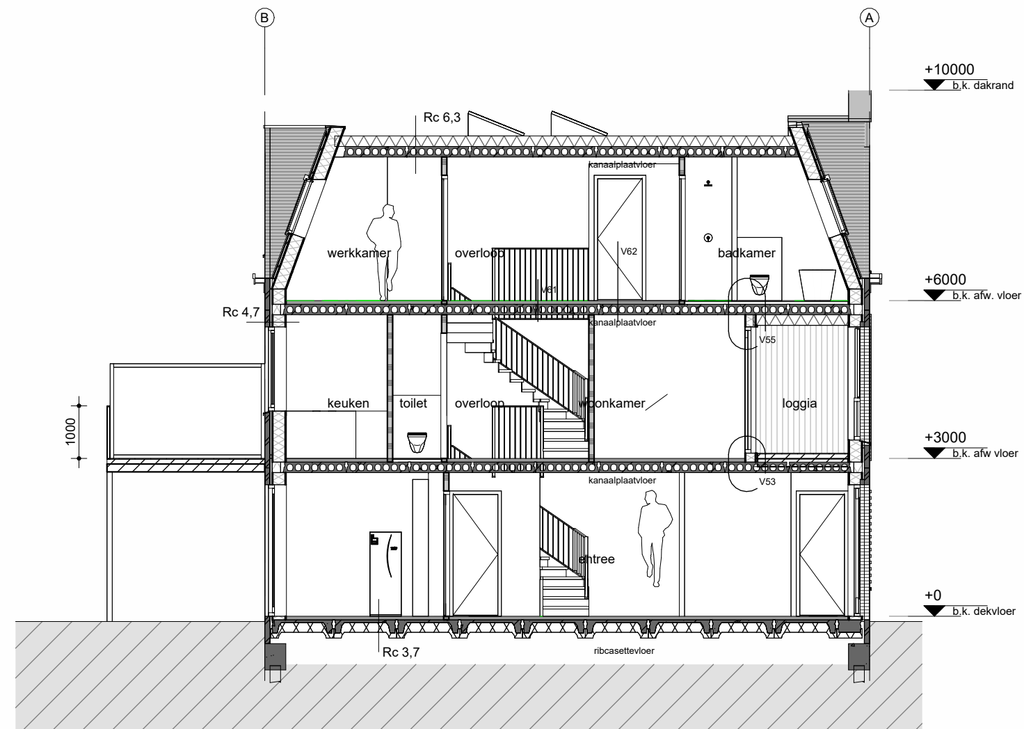
Doorsnede B-B
