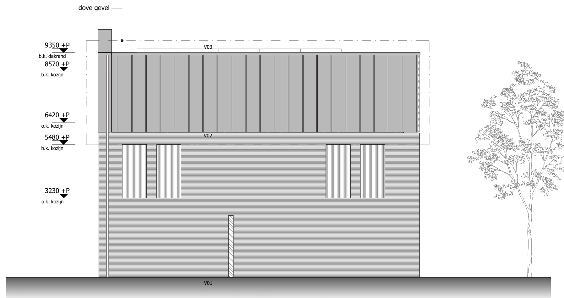
Rechter zijgevel
