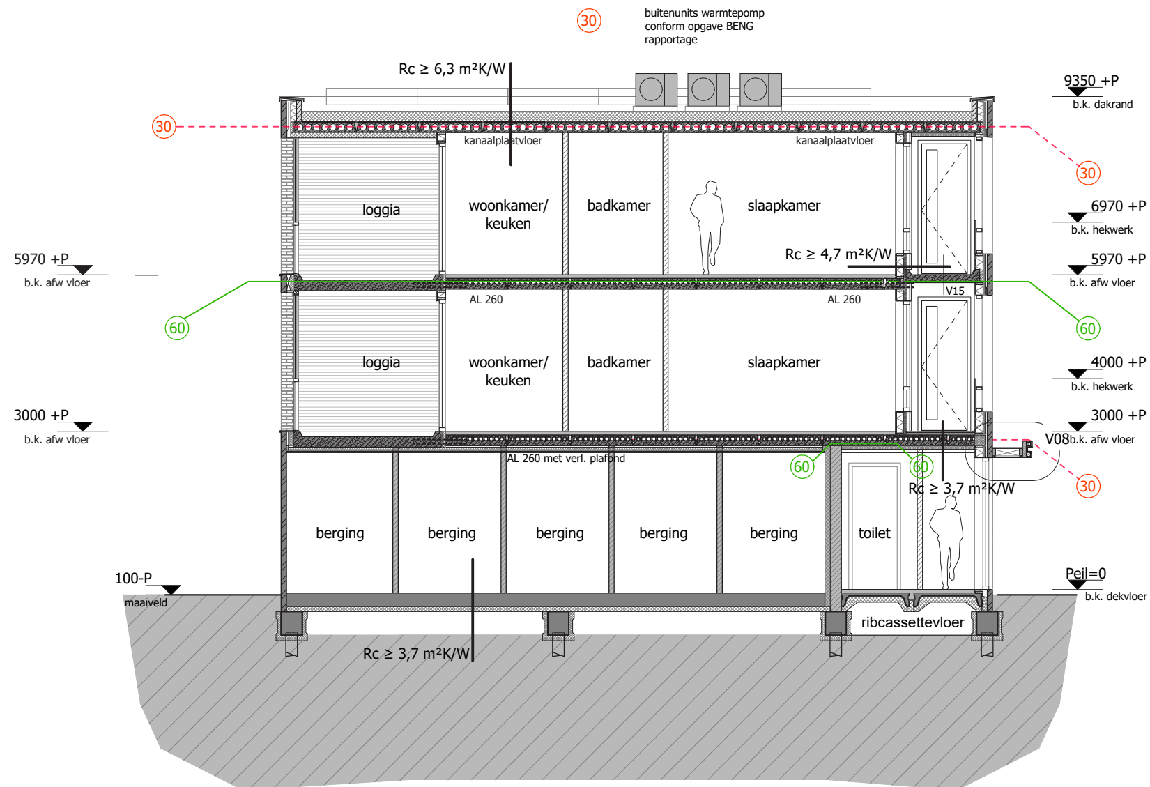
Doorsnede B-B
