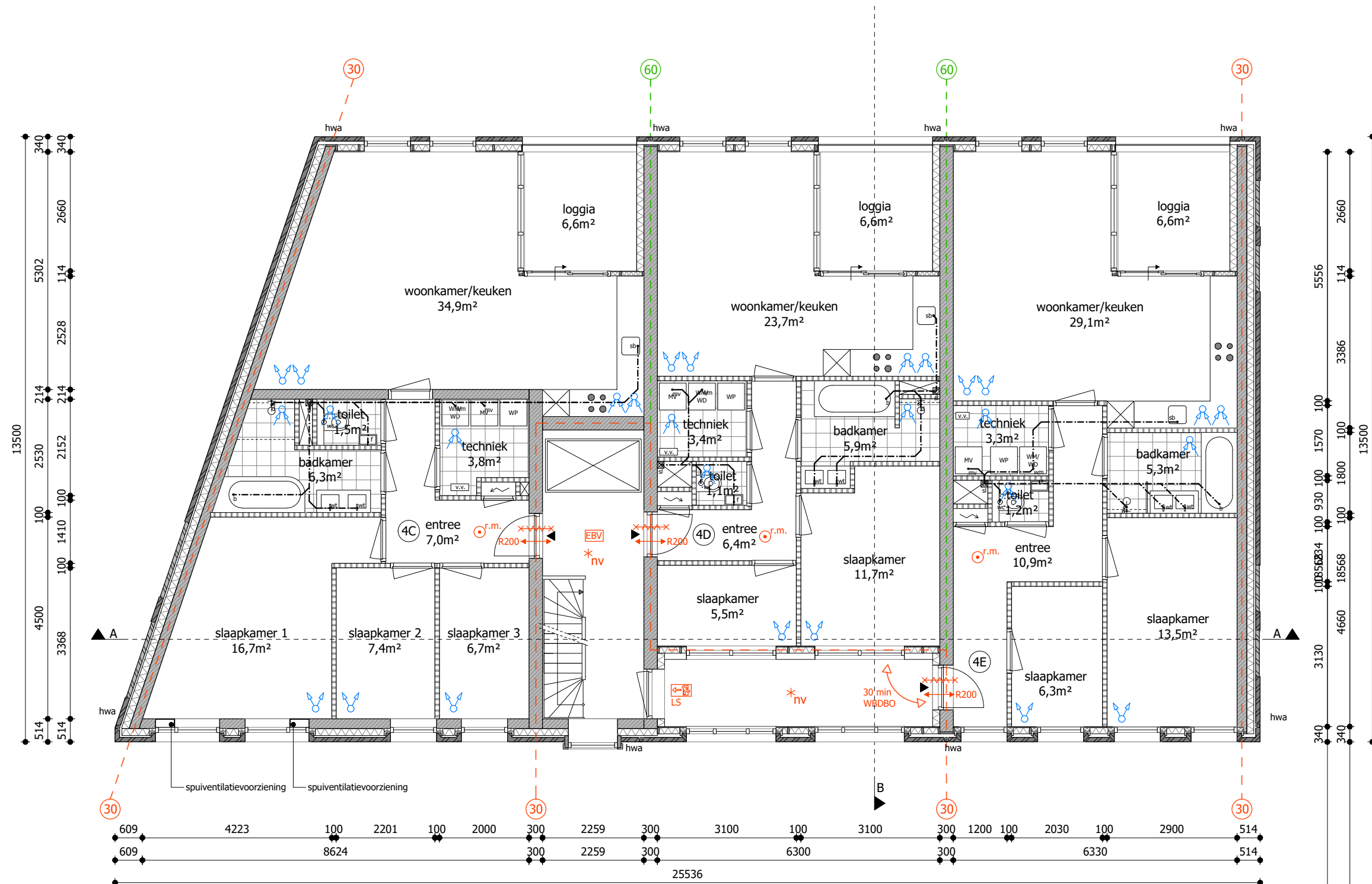
Eerste verdieping
