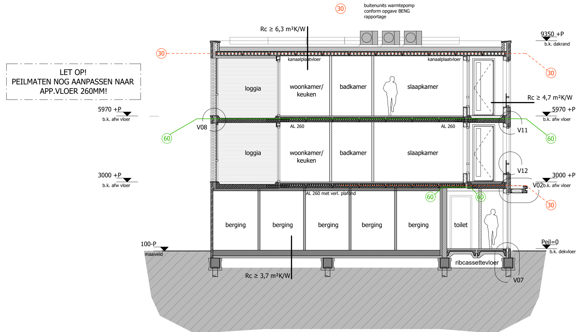
Doorsnede B-B
